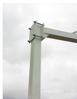
Amarre doble pletina vuelo
